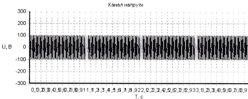
Рисунок 1 — Складений сигнал для першої перевірки: помаранчеві ділянки — конвертований сигнал, червоні — гармоніка 50 Гц.
