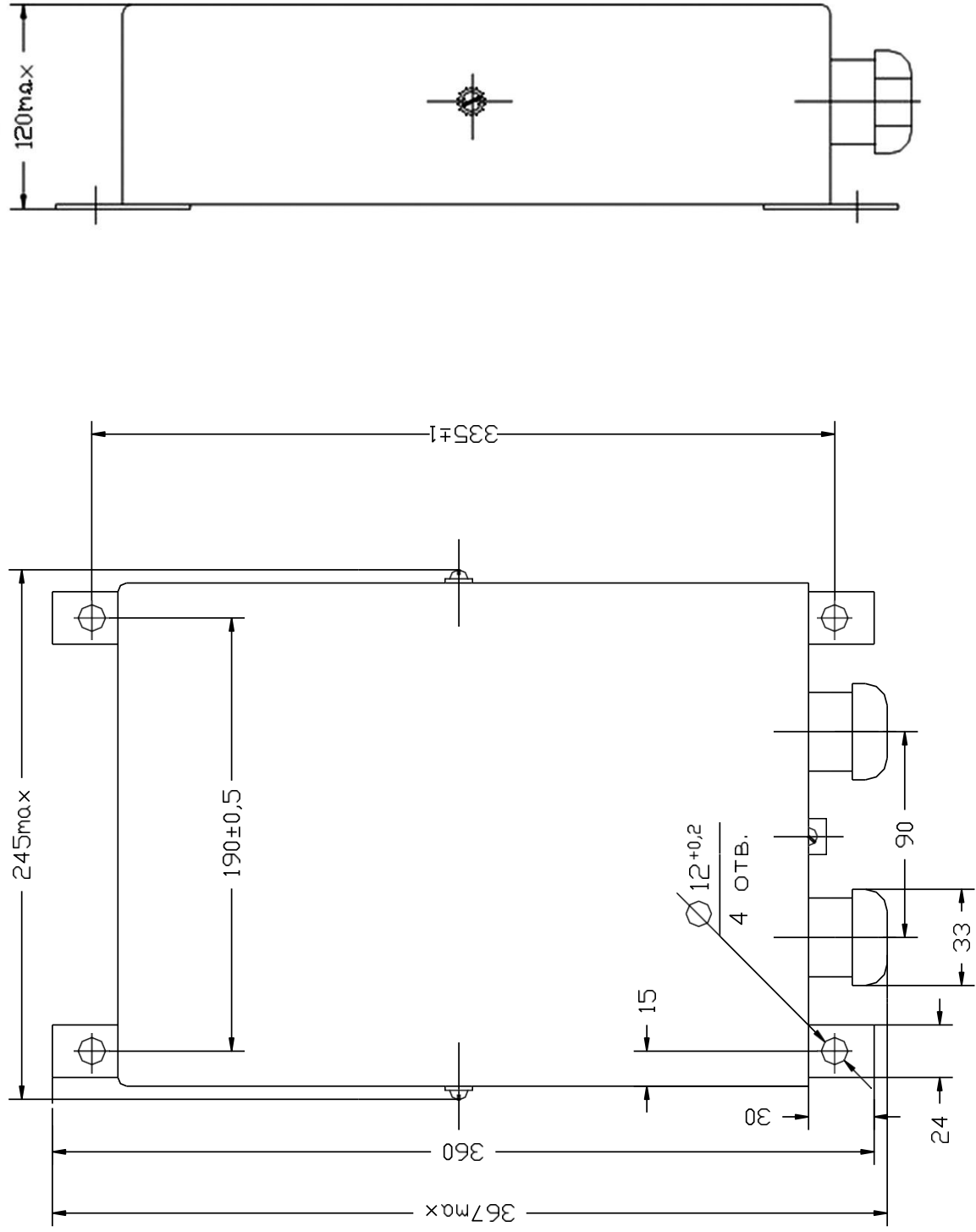
Габаритные и установочные размеры.
